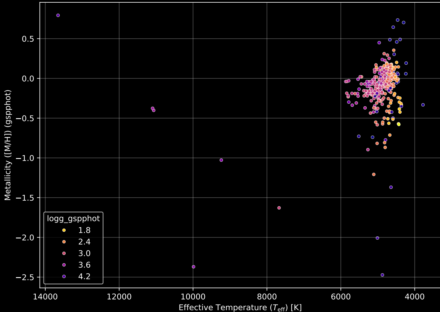
APOGEE DR17 Field: [281-06] Stellar Population Parameters (n= 361)
