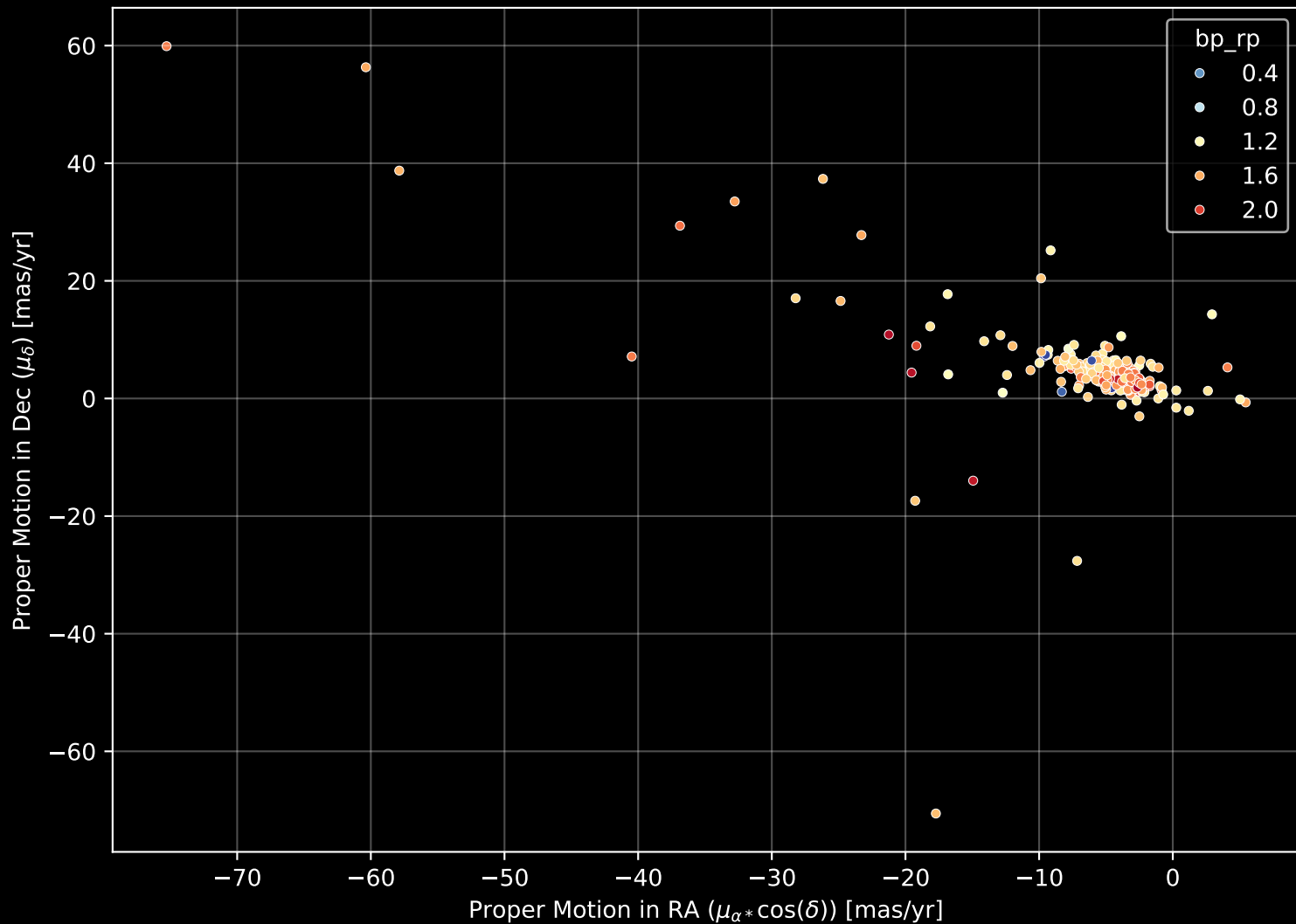
APOGEE DR17 Field: [281-06] Proper Motion Diagram (n= 361)
