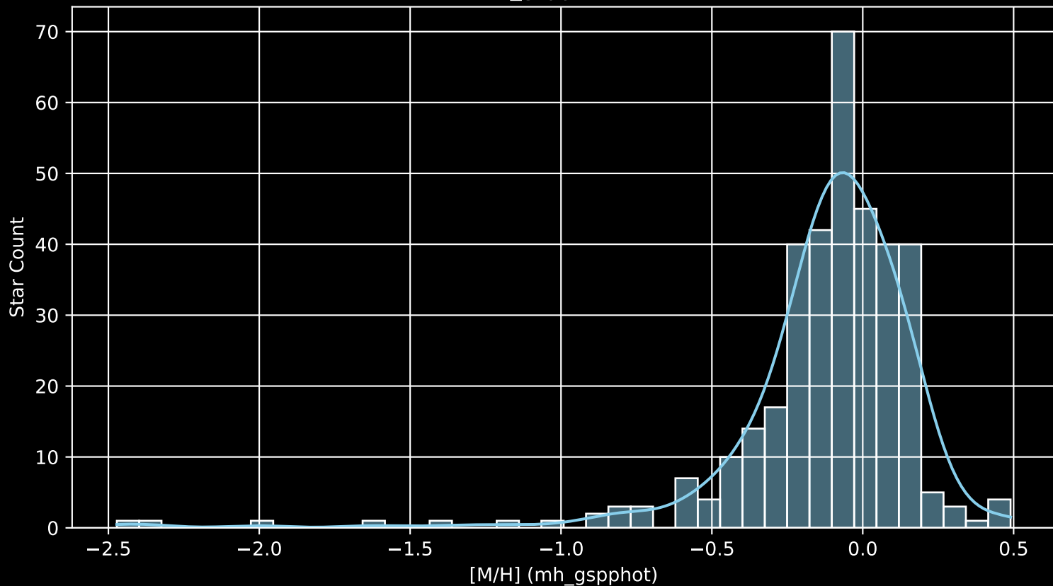
APOGEE DR17 Field: [281-06 [M/H] (mh_gspphot) (n= 357)
